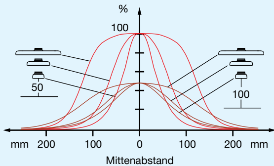
Bild 14: Räumliche Strahlungsverteilung
