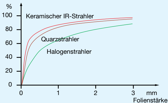
Bild 20: Absorption bei transparenten Folien
