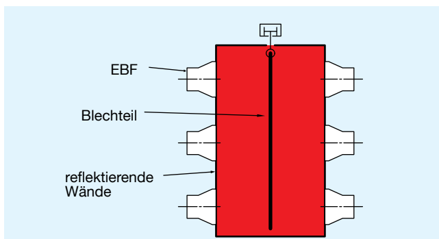
Bild 11: Strahlungstunnel mit mehreren EBF-Systemen
