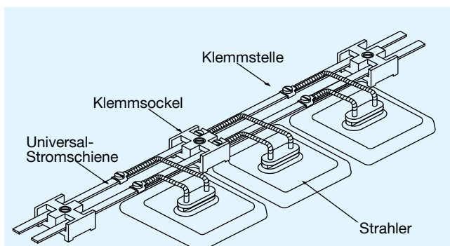
Bild 13: Schienenverdrahtung
