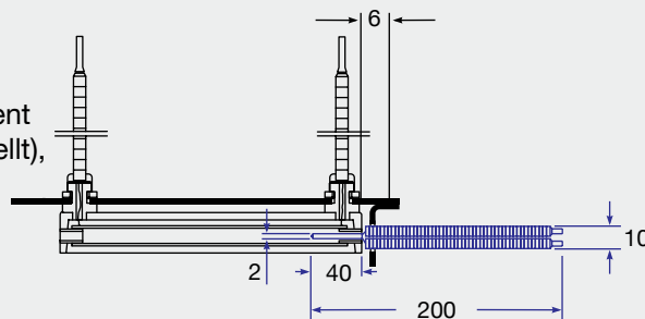
Bild 60: Einbaumaße und Strahlerabmessungen ( ) in mm
