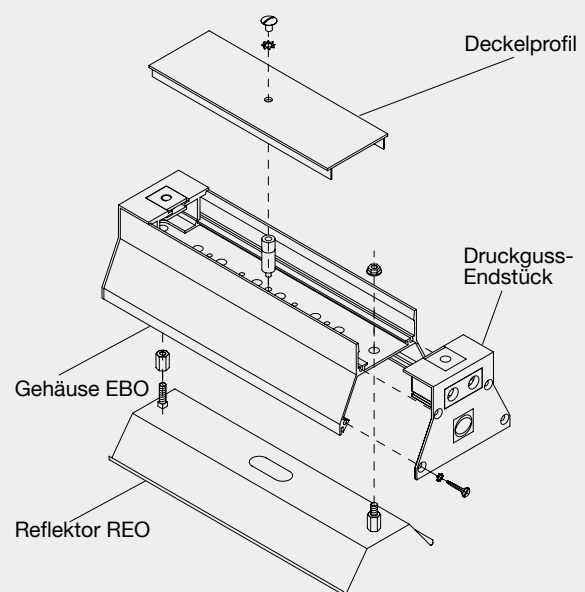
Bild 97: Beispiel für die Anordnung von Metallteilen anhand eines Gehäuses EBO mit Reflektor REO
