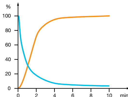
Bild 46: Strahlungsleistungen Aufheizen: rote Kurve Abkühlen: blaue Kurve
