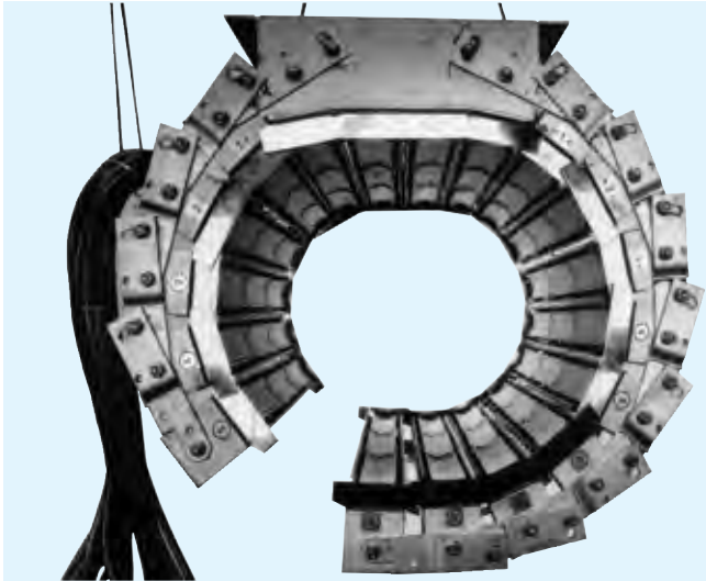
Bild 28: Heizkopf zur Erwärmung von GFK-Rohren
