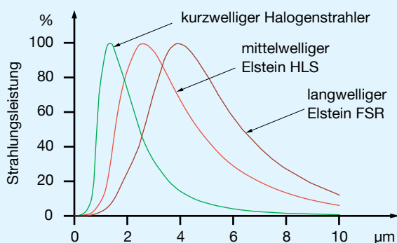
Bild 3: Spektrale Strahlungsleistung
