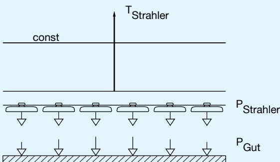
Bild 15: Leistung am Gut bei konstanter Strahlerleistung
