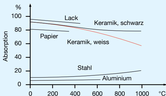
Bild 5: Absorption verschiedener Werkstoffe
