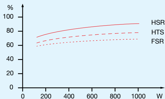
Bild 21: Wirkungsgrade abhängig von der Leistung
