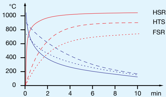
Bild 18: Aufheiz- und Abkühlverhalten
