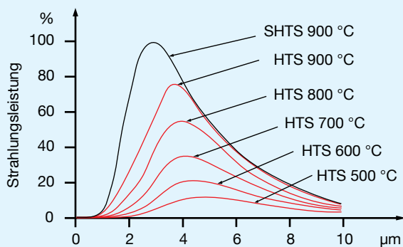
Bild 4: Spektrale Strahlungsleistung Elstein Strahler
