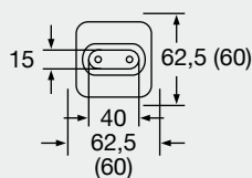
Bild 36: Einbaumaße und Strahlerabmessungen ( ) in mm
