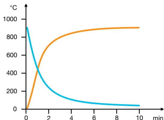
Bild 57: Strahlertemperaturen Aufheizen: rote Kurve Abkühlen: blaue Kurve
