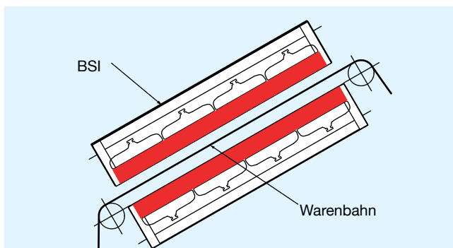
Bild 12: Beheizung einer Warenbahn mit 2 BSI-Systemen
