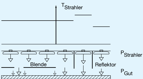
Bild 17: Leistungsanpassung mit Reflektor und Blende
