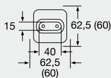
Bild 32: Einbaumaße und Strahlerabmessungen ( ) in mm
