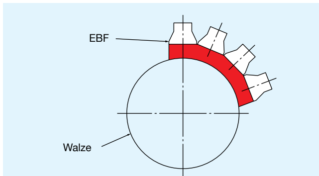
Bild 10: Walzenbeheizung mit dem EBF-System
